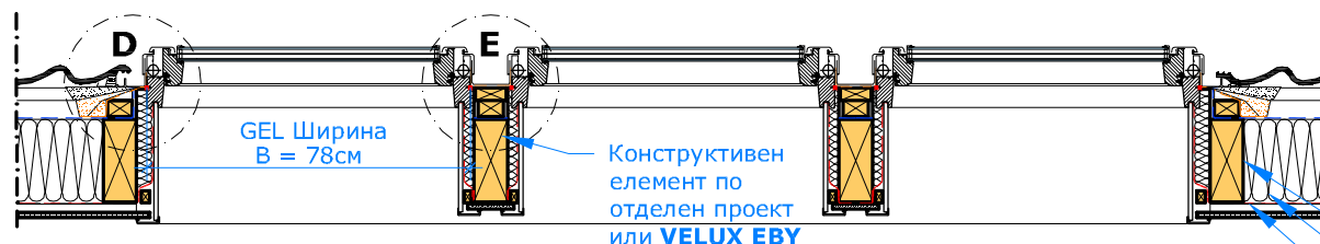
Разрез В-В M10
