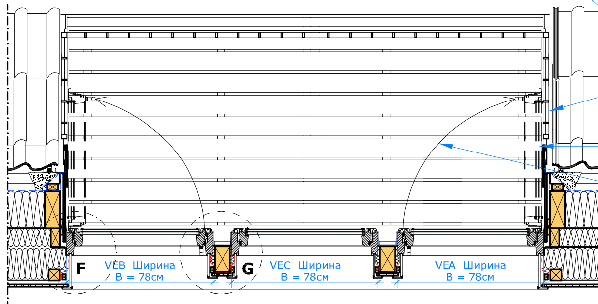
Разрез С-С M10
